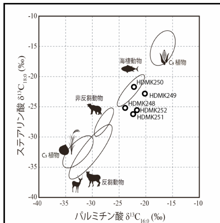
図 2. \delta^{13}\text{C}_{16:0} と \delta^{13}\text{C}_{18:0} の分子レベル炭素同位体組成結果を、現生日本産生物データ (堀内ほか 2014, Horiuchi et al.2014, 吉田ほか 2018) と比較した図
